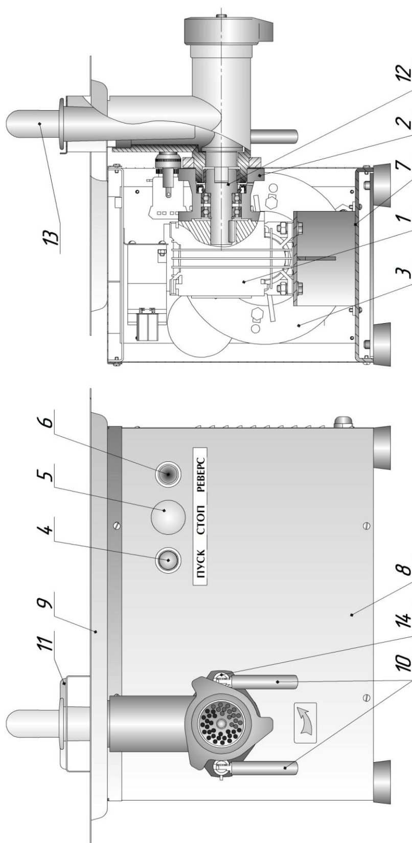
Рисунок - 3 Мясорубка М-80С
