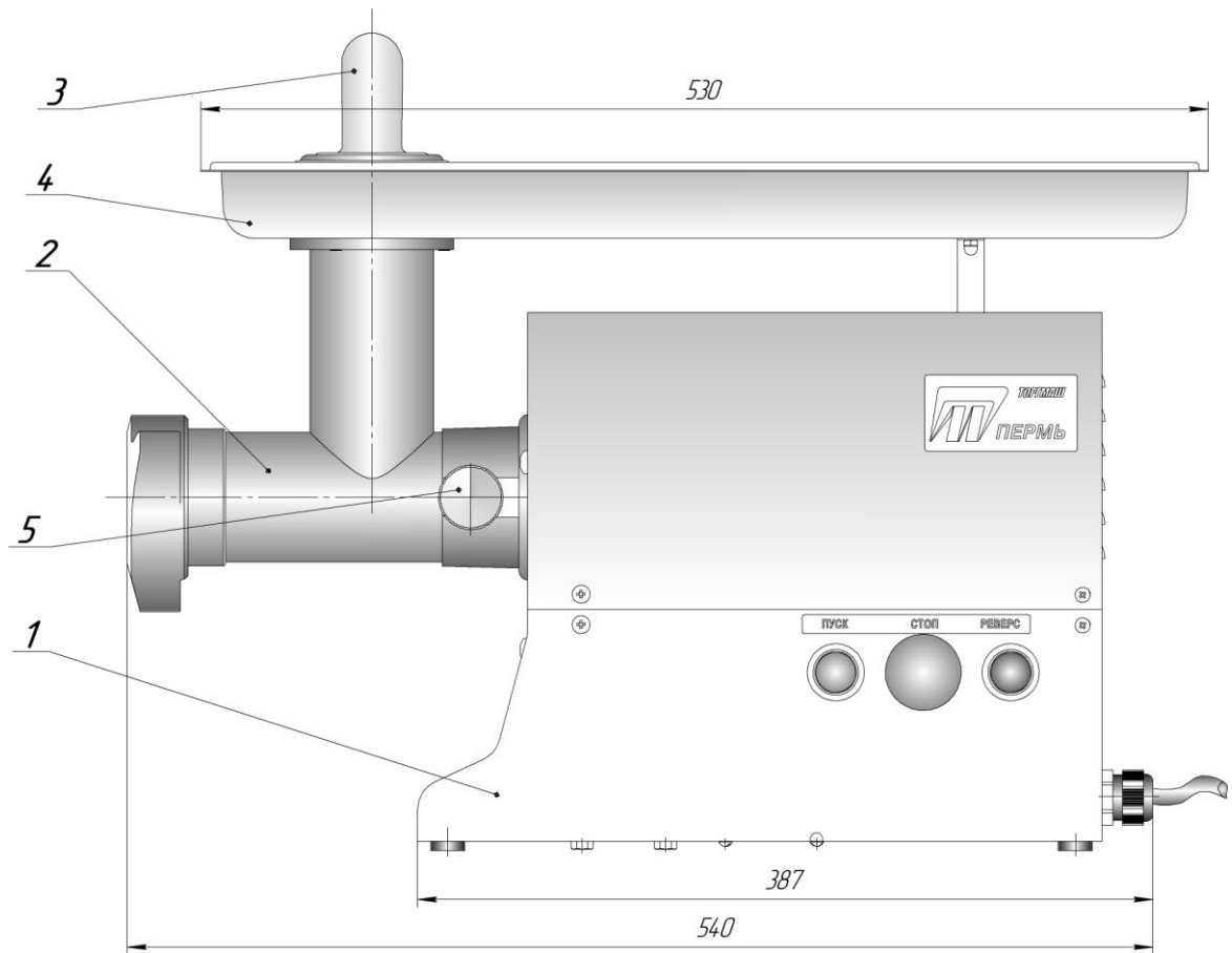
Рисунок 1 – Мясорубка М-80М/220
